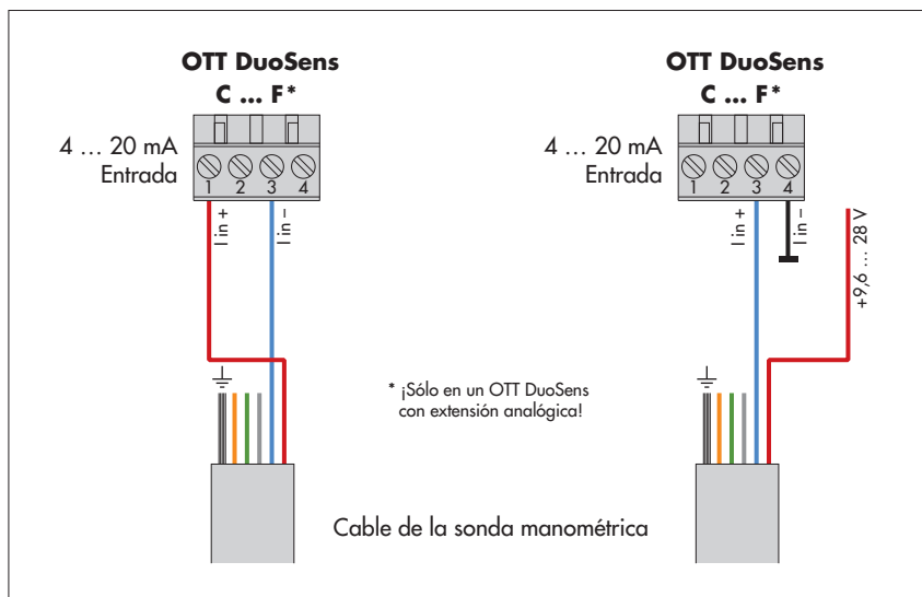
Fig. 13: Conexión del OTT PLS a OTT DuoSens mediante la interfaz de 4 ... 20 mA.
