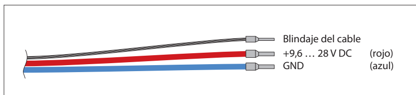
Fig. 5: Conectores utilizados con el empleo de la interfaz de 4 ... 20 mA. Si debe configurarse la OTT PLS por medio de la interfaz RS-485, se necesitará además el conector verde y naranja.
