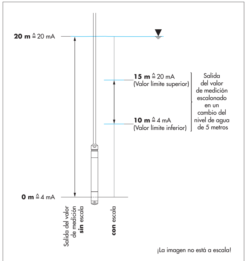
Fig. 7: Escalonado de la salida del valor de medición de la interfaz de 4 ... 20 mA a un margen de medición menor.
