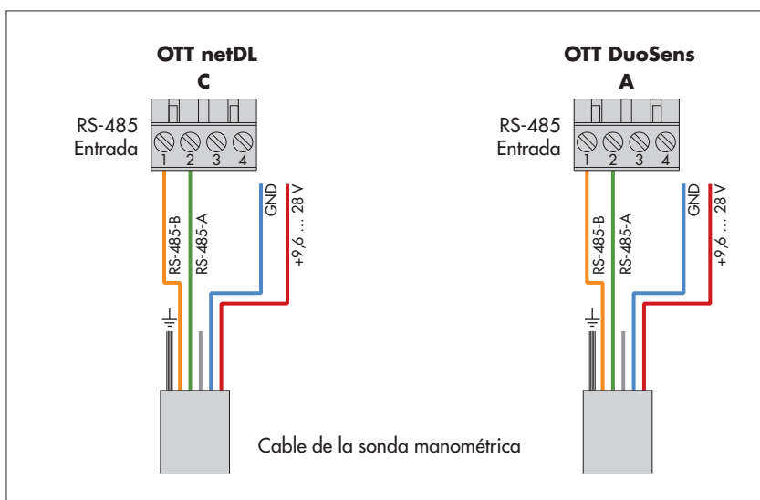
Fig. 10: Conexión de OTT PLS a OTT netDL o a OTT DuoSens mediante la interfaz RS-485 (protocolo SDI-12).
