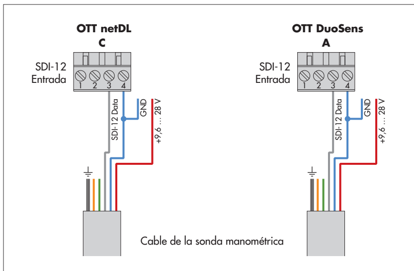
Fig. 9: Conexión de OTT PLS a OTT netDL o a OTT DuoSens mediante la interfaz SDI-12.
