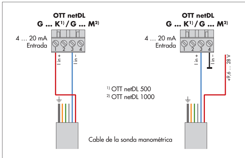
Fig. 12: Conexión del OTT PLS a OTT netDL mediante la interfaz de 4 ... 20 mA.
