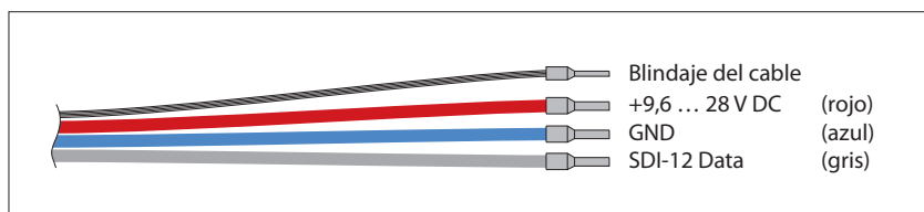
Fig. 4: Conectores utilizados con el empleo de la interfaz SDI-12.
