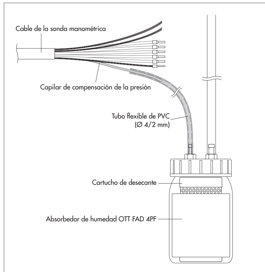
Fig. 16: Instalación del absorbedor de humedad OTT FAD 4PF.
